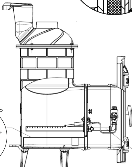
Колосниковое дно
