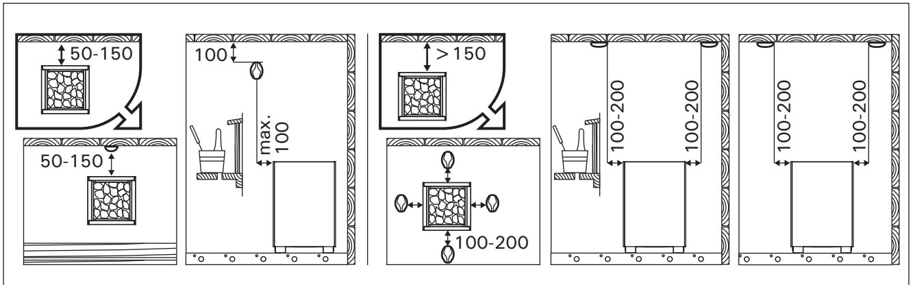
Figure 5. Installing the sensor (all dimensions in millimeters) Abbildung 5. Installation der Fühler (alle Abmessungen in Millimetern)
