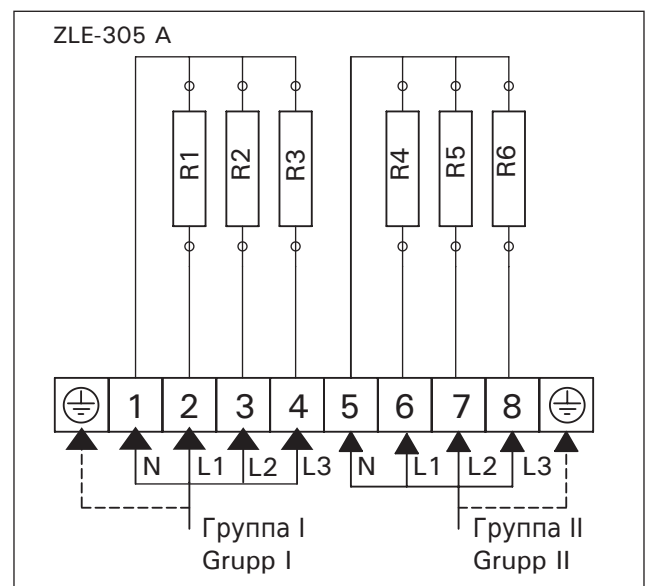
Рисунок 9. Электромонтаж каменки, установленной в качестве групповой Joonis 9. Elektrihendused kahes grupis
