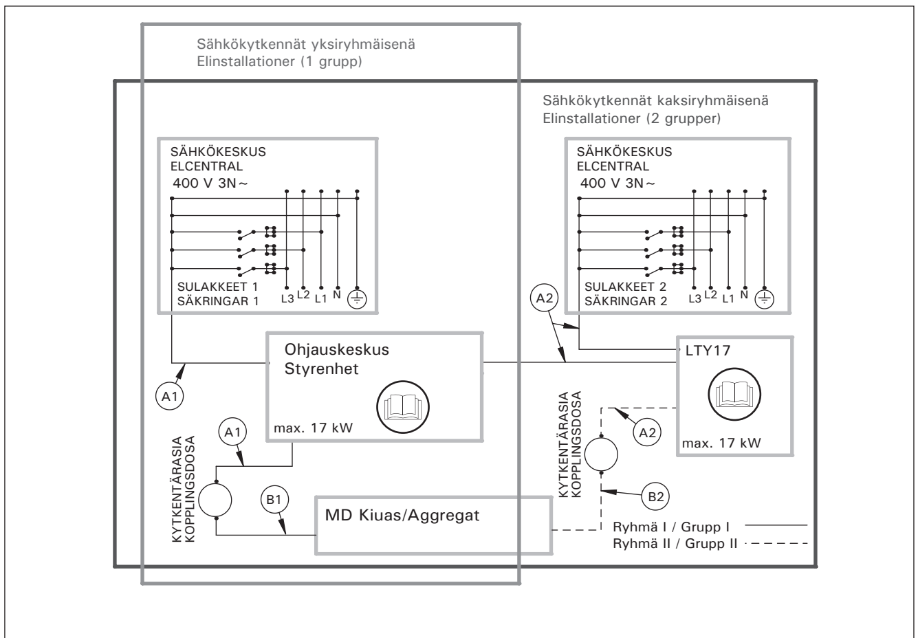
Kuva 11. Ohjauskeskuksen ja MD-kiukaan sähkökytkennät Bild 11. Elinstallationer av styrenhet och MD-aggregat
