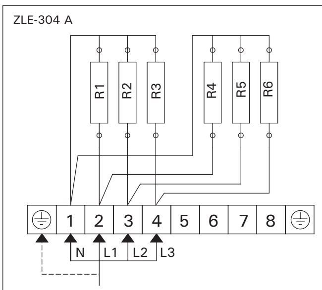
Рисунок 8. Электромонтаж Joonis 8. Elektrihendused
