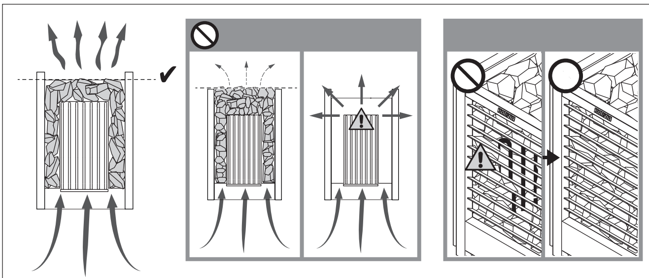
Рисунок 1. Укладка камней
