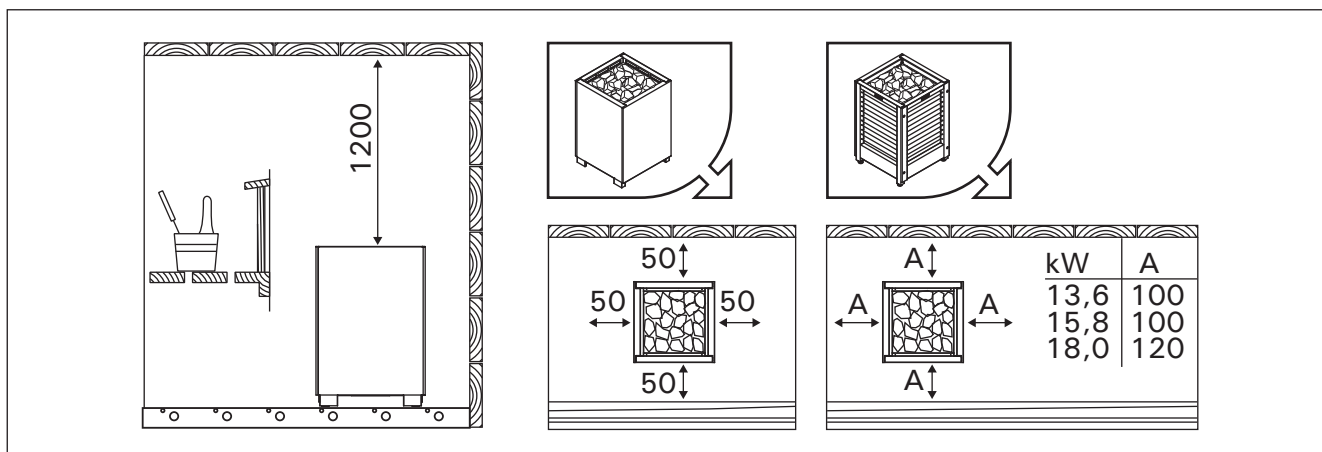
Kuva 4. Kiukaan minimisuojaetäisyydet (mitat millimetreinä)
