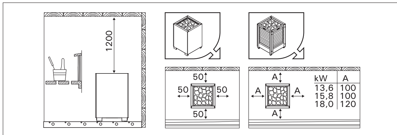
Рисунок 4. Расстояния безопасности (все размеры приведены в миллиметрах) Joonis 4. Kerise miinimum ohutuskaugused (kõik mõõtmised millimeetrites)
