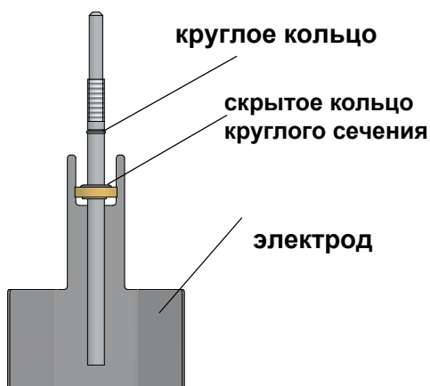
Двойное уплотнение электродов для парового цилиндра CY45/2 (SLE45/65)
